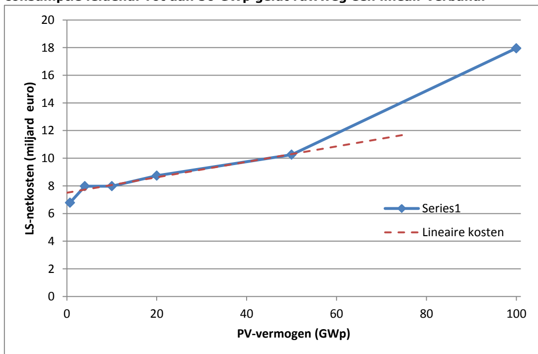
Figuur 23 Investeringskosten (eenmalig) van het laagspanningsnet als functie van de penetratiegraad van PV in Nederland zonder curtailment. Tot aan 10 GWp is niet PV, maar de consumptie leidend. Tot aan 50 GWp geldt ruwweg een lineair verband.
