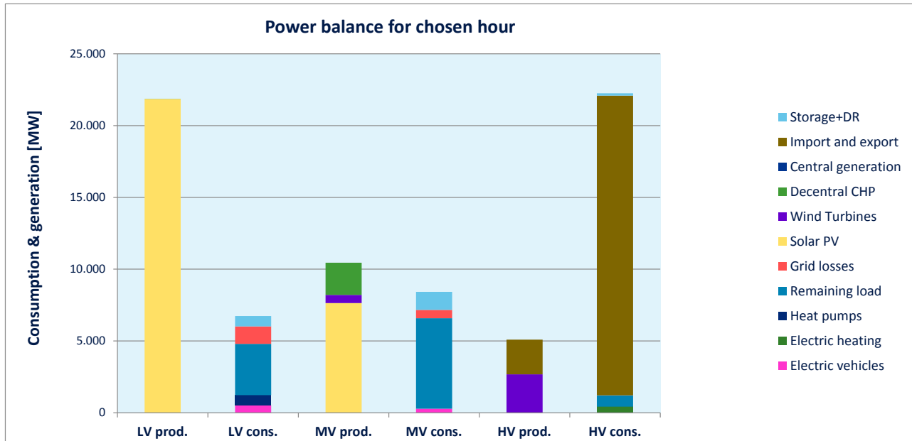
Figuur 20 De vermogensbalans in Nederland in het uur met de hoogste PV-productie voor een opgesteld PV-vermogen van 150 GWp met 75% curtailment in Nederland, met 20% demand response en 50% penetratie van warmtepompen, elektrische verwarming en EV's
