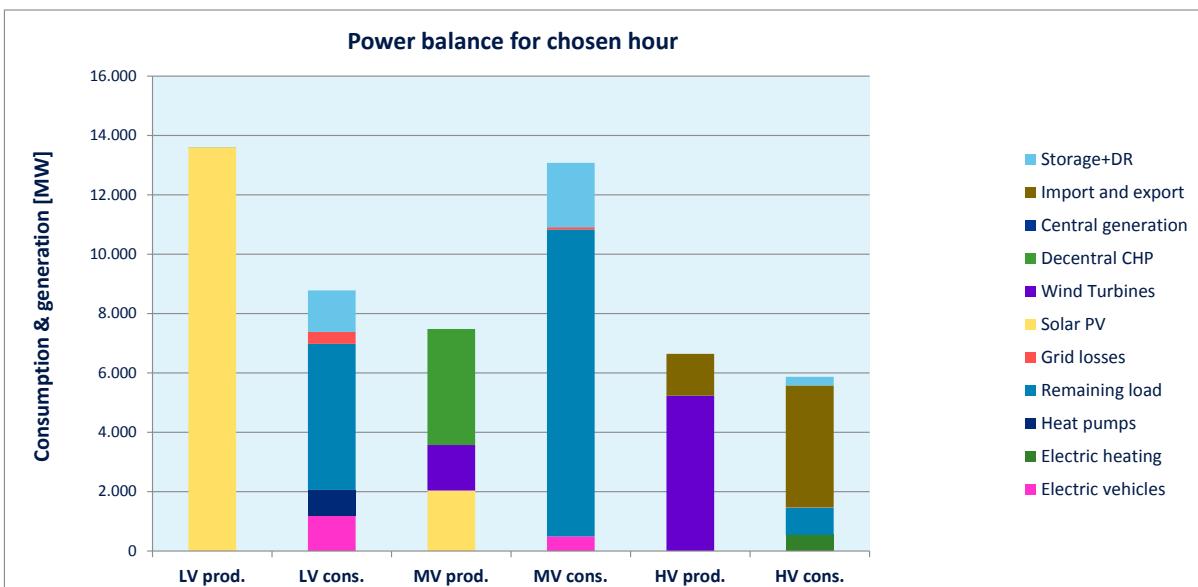
Figuur 15 De vermogensbalans in Nederland in het uur met de hoogste PV-productie voor een opgesteld PV-vermogen van 20 GWp in Nederland, met een combinatie van demand response (20%), elektrische voertuigen (50%), warmtepompen (45%) en elektrische verwarming (55%)
