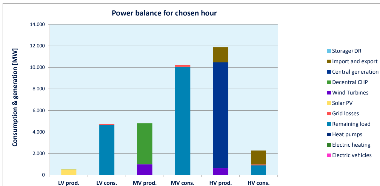
Figuur 4 De vermogensbalans in Nederland in het uur met de hoogste PV-productie voor een opgesteld vermogen van 700 MWp in Nederland
