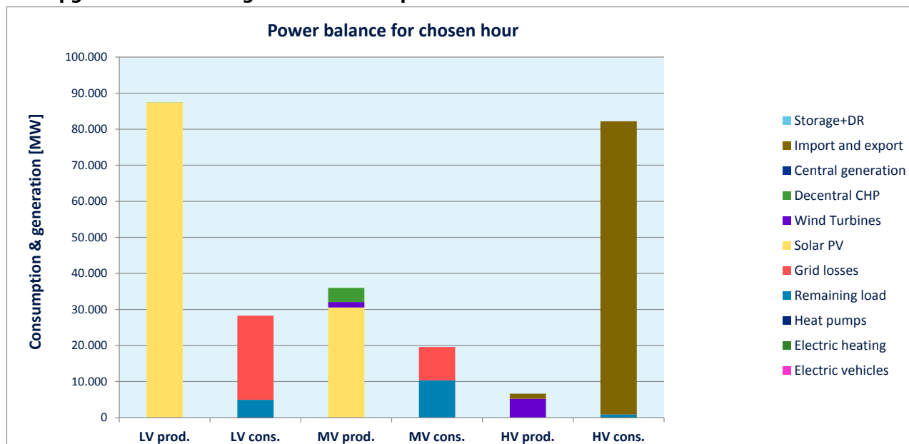
Figuur 17 De vermogensbalans in Nederland in het uur met de hoogste PV-productie voor een opgesteld PV-vermogen van 150 GWp in Nederland
